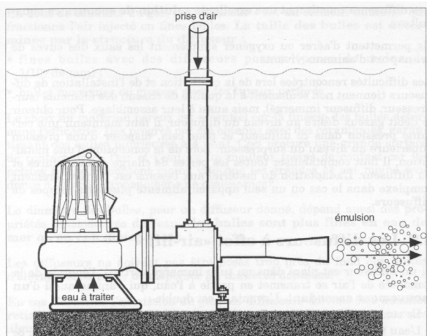
Fig. 19 – Schéma d'un hydro-éjecteur (d'après notice Flygt).
