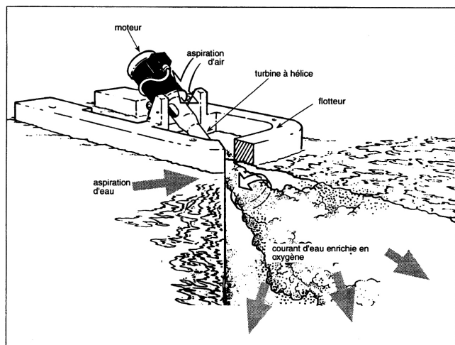
Fig. 18C – Schéma d'une pompe émulseuse (d'après notice Aire-O 2 ®).
