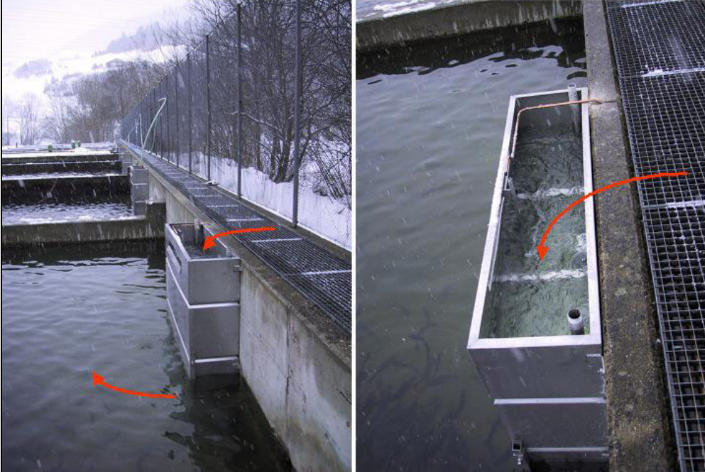
La plate-forme à jets gravitaire en inox
